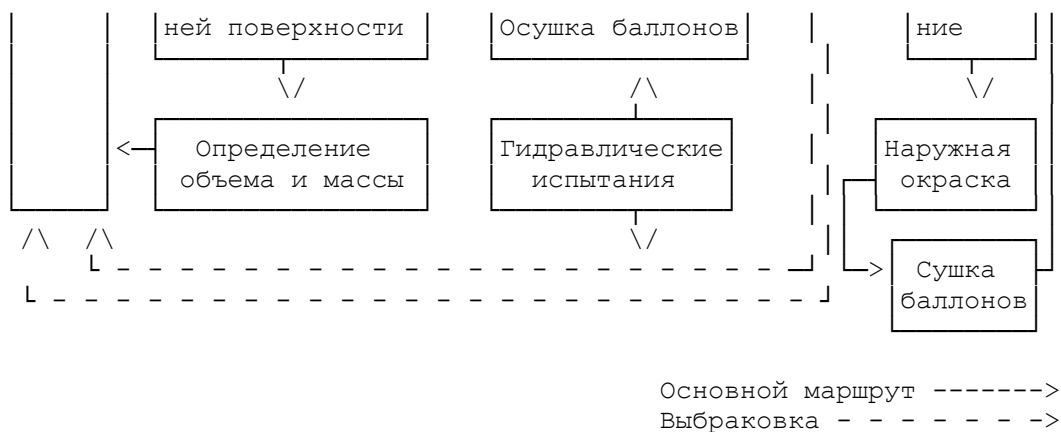
Рис. 10.2. Технологическая схема освидетельствования баллонов
