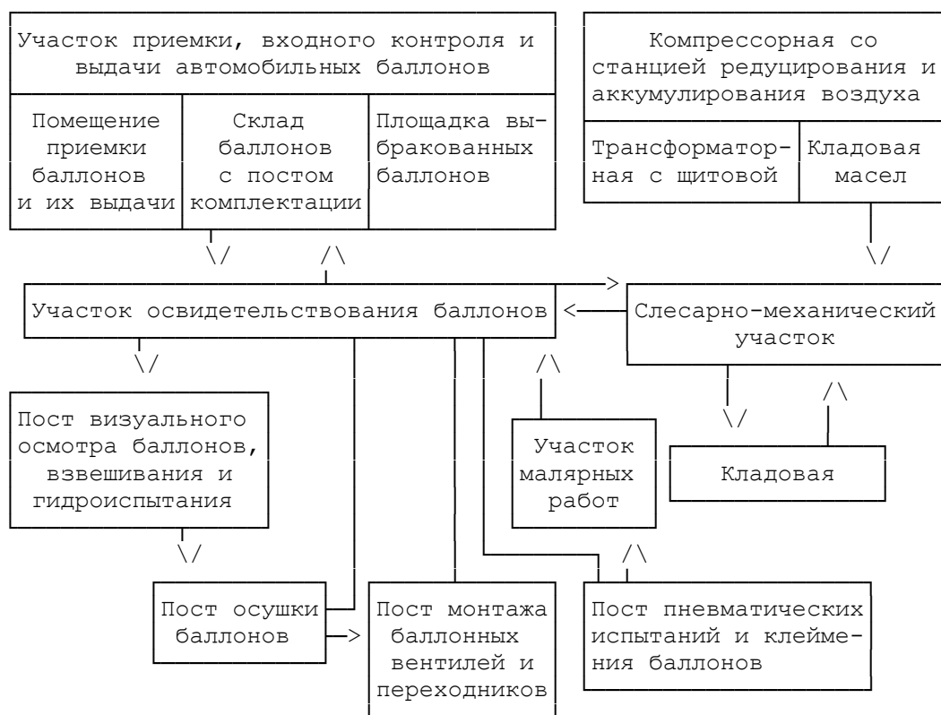
Рис. 10.1. Схема пунктов освидетельствования баллонов
