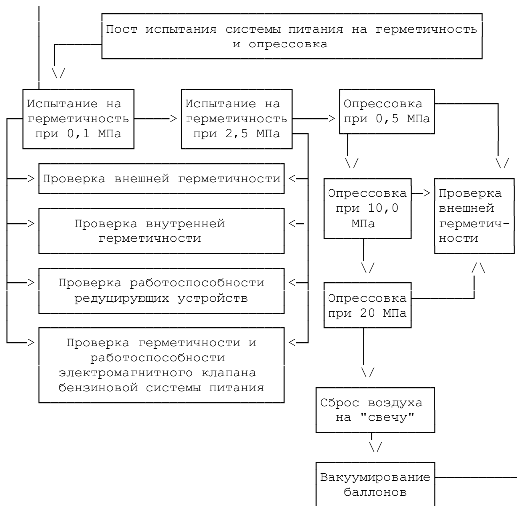
Рис. 9.1. Технологическая схема испытаний автомобилей, работающих на КПП
