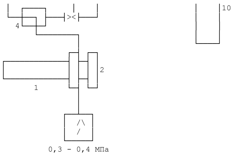
Рис. 5.4. Схема пневматической установки по выпуску газа и дегазации газовых баллонов на автомобиле в условиях АТП
