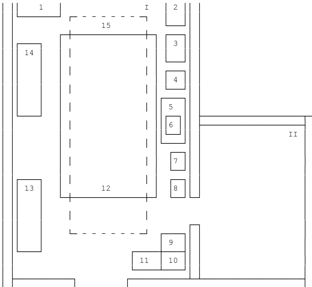
Рис. 5.5. Участок ТО и ТР газобаллонных автомобилей
