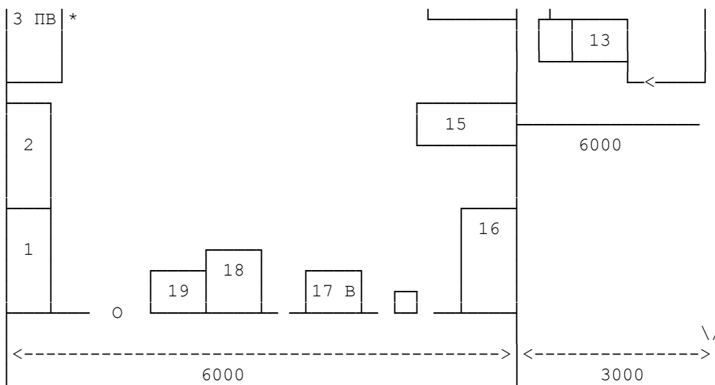
Рис. 5.6. Примерная планировка цеха ТО и ТР газовой аппаратуры в АТП
